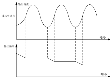
图6-24 过压失速功能
