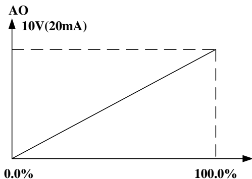
图6-13 给定量与模拟量输出的对应关系
