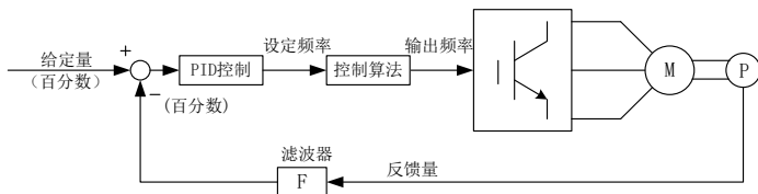
图6-21 过程PID原理框图
