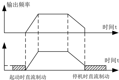
图6-4 直流制动时间表
