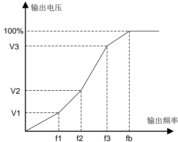
图 6-7 V/F 曲线示意图
