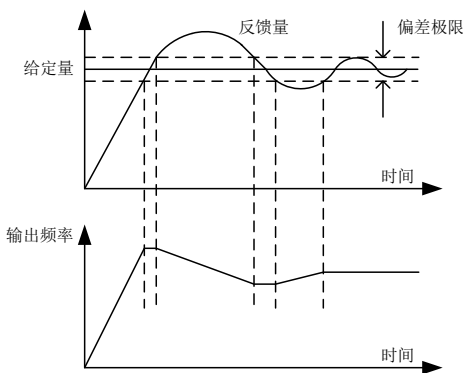
图6-22 偏差极限与输出频率的对应关系
