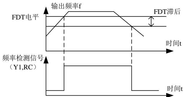
图6-17 FDT电平示意图
