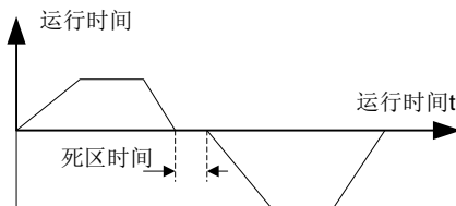
图6-5 正反转死区时间指示
