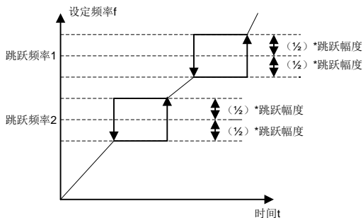
图 6-6 跳跃频率指示图
