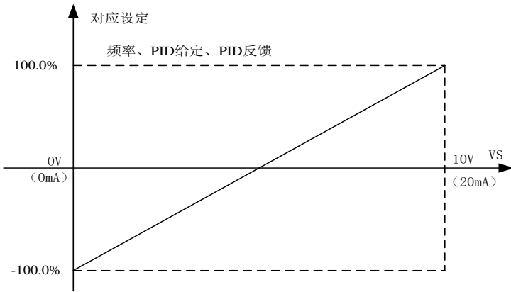
图6-12 模拟给定与设定量的对应关系
