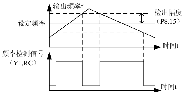
图6-18 频率到达检出幅值示意图
