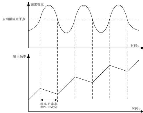
图6-25 限流保护功能示意图
